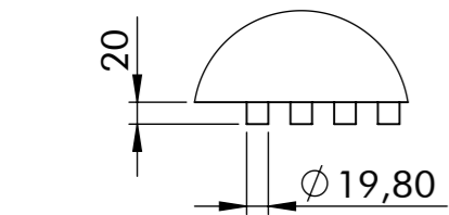
DETAIL C MAßSTAB 2 : 15
